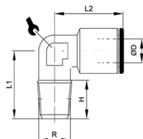
THREADED ELBOW ADAPTOR TAPER / ÉQUERRE MALE CONIQUE FIXE / GOMITO MASCHIO CONICO FISSO
