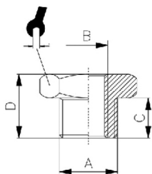
REDUCER PARALLEL / RÉDUCTION CYLINDRIQUE / RIDUZIONE CILINDRICA
