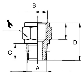
EXTENSION TAPER / RÉDUCTION CONIQUE / PROLUNGA RIDUZIONE CONICA
